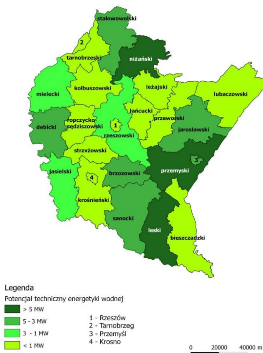
Rysunek 11 Potencjał techniczny energetyki wodnej w województwie podkarpackim
