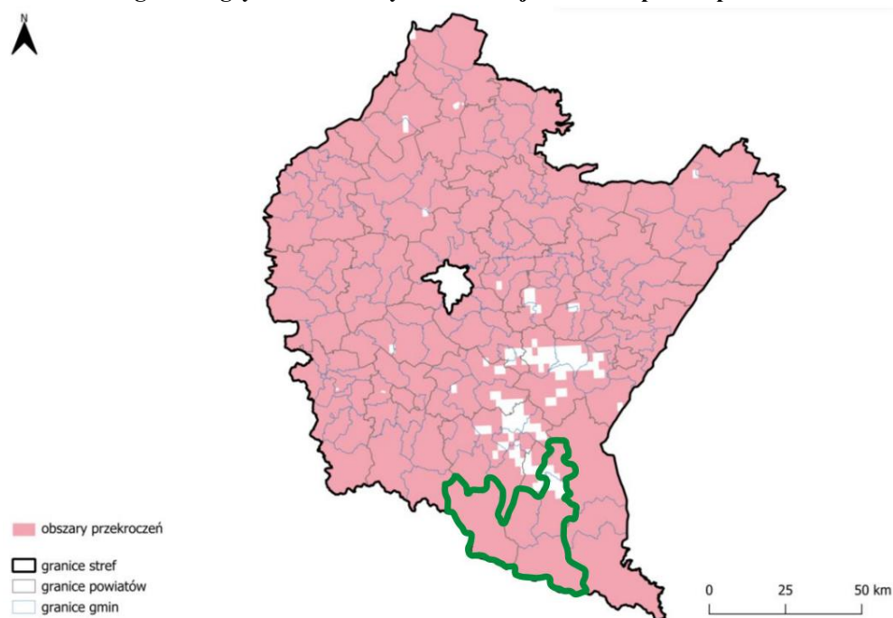
Mapa 19 Zasięg obszaru przekroczenia poziomu celu długoterminowego (wskaźnika AOT40) dla O 3 ustanowionego ze względu na ochronę roślin w województwie podkarpackim w 2024 r.
